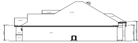
RIGHT ELEVATION SCALE: 1/8"=1'-0"
